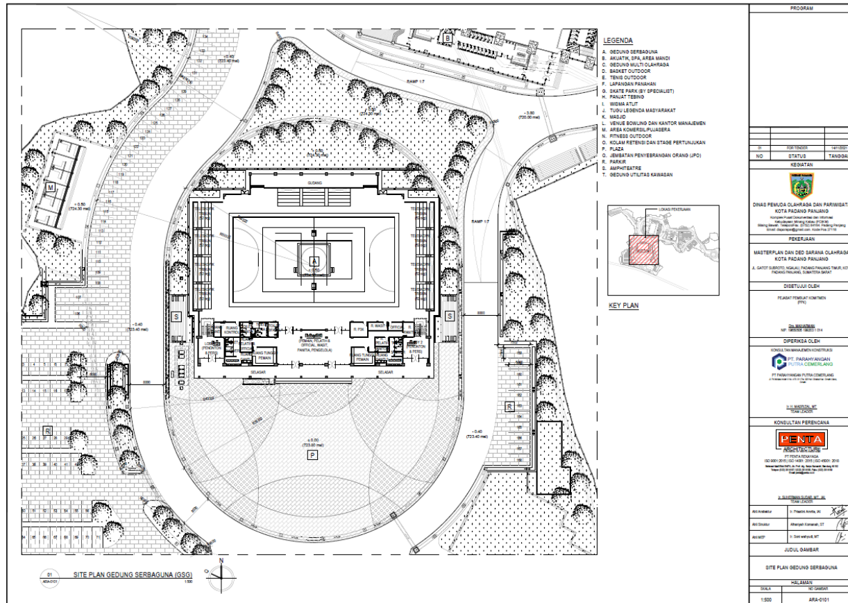
Site Plan Gedung Serba Guna
